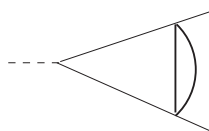
V4l2M2m
