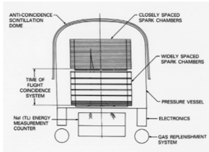
Abbildung 5.5: Schema der EGRET-Apparatur.
