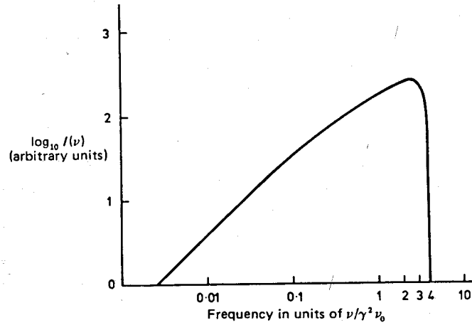
Abbildung 5.15: Energiespektrum der Photonen nach inverser Compton-Streuung ( E_\gamma = h\nu ).
