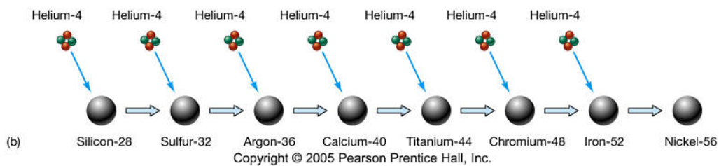
Abbildung 6.11: Schematische Darstellung der Produktion schwerer Elemente.
