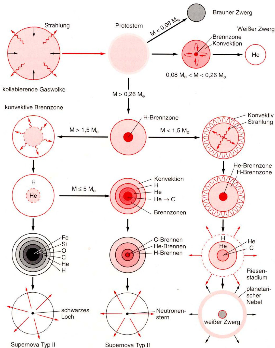
Abbildung 6.13: Entwicklungswege der Sterne in Abhängigkeit von ihrer Masse.
