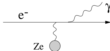
Abbildung 3.14: Bremsstrahlung bei der Rutherford-Streuung im Coulomb-Feld eines Kerns.
