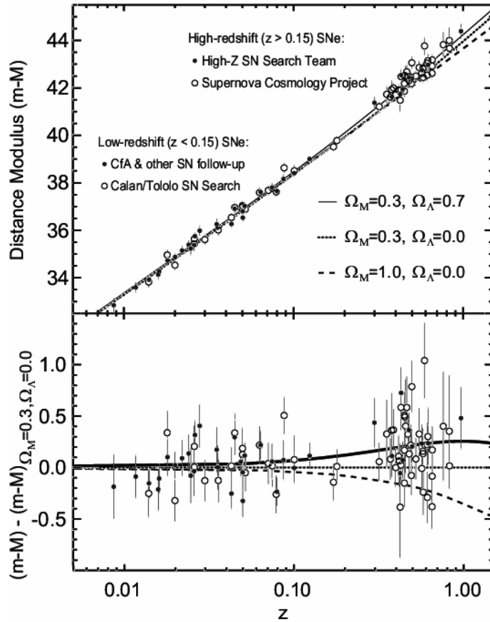
Abbildung 6.18: Die Leuchtkraft von Supernovae Ia als Maß für die Entfernung aufgetragen gegen die Rotverschiebung legt eine Abweichung vom Hubble-Gesetz nahe. Die Daten sind am besten mit einer kosmologischen Konstante entsprechend \Omega_\Lambda \approx 0.7 verträglich.
