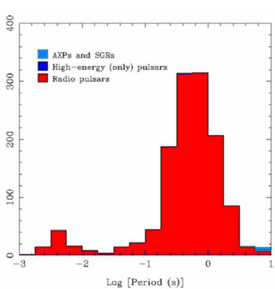
Abbildung 6.20: Verteilung der Perioden der beobachteten Pulsare.
