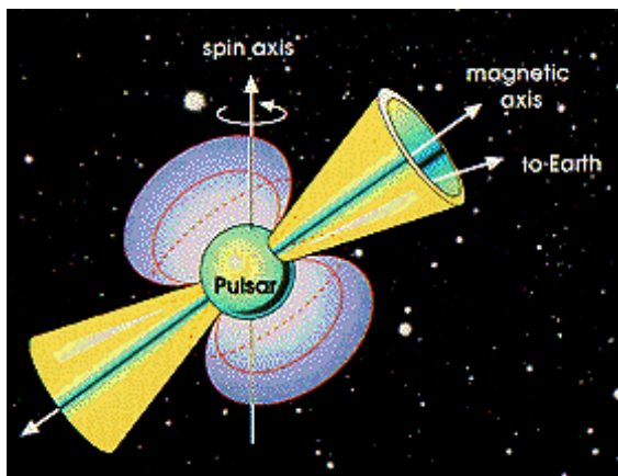
Abbildung 6.19: Neutronenstern, bei dem die Rotationsachse und die Dipolachse des Magnetfeldes gegeneinander geneigt sind.
