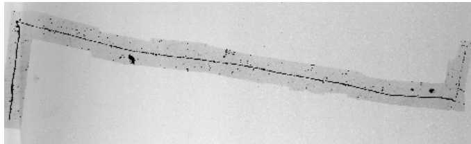
Abbildung 3.2: Teilchenspuren aufgenommen während eines Ballonfluges in einer Photoemulsion: Zerfall eines Pions in ein Myon, das dann in ein Elektron zerfällt ( \pi - \mu - e - Zerfall).
