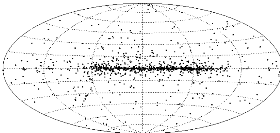
Abbildung 6.21: Verteilung der bekannten Pulsare.
