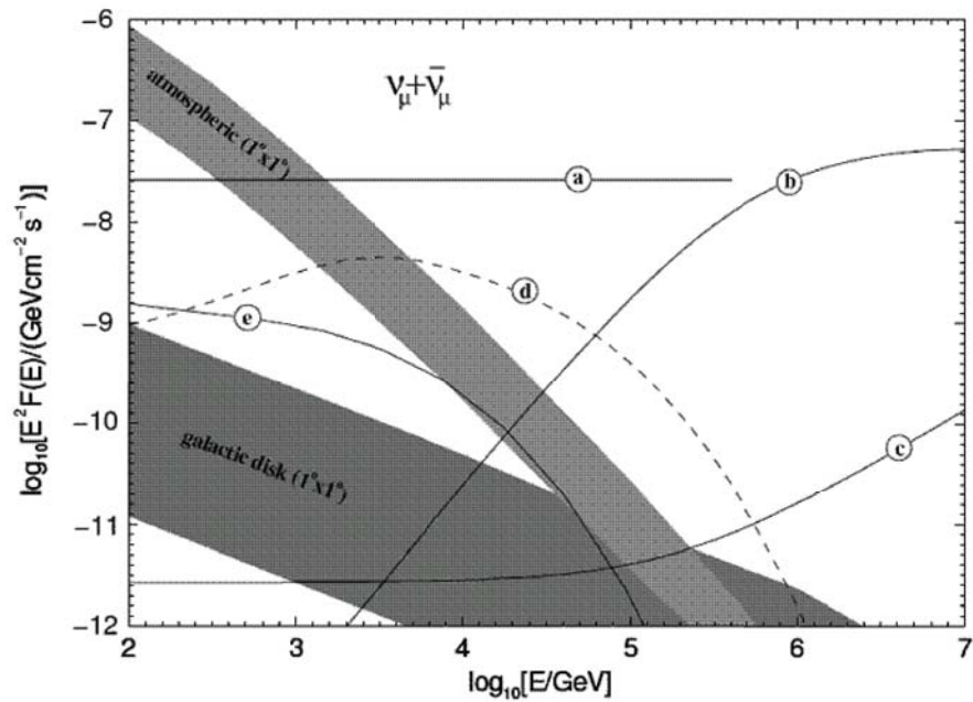
Abbildung 4.13: Vorhergesagte Neutrinoemissionen als Funktion der Energie verglichen mit dem Spektrum atmosphärischer Neutrinos (schattiertes Band): a)-c) Verschiedene Vorhersagen für AGN 3C273, d) Neutrinoemission vom Krebsnebel, e) Neutrinoemission vom SN-Rest Cassiopeia A. Das flachere der schattierten Bänder stellt die Vorhersage für Neutrinos aus Wechselwirkungen von Kosmischer Strahlung in der galaktischen Scheibe dar.
