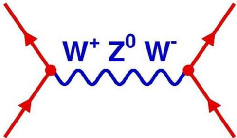
schwache Kraft
