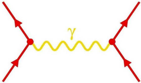
elektromagn. Kraft
